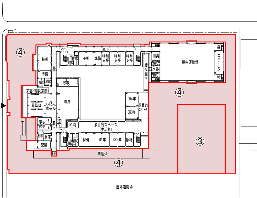
配置・1階計画図
