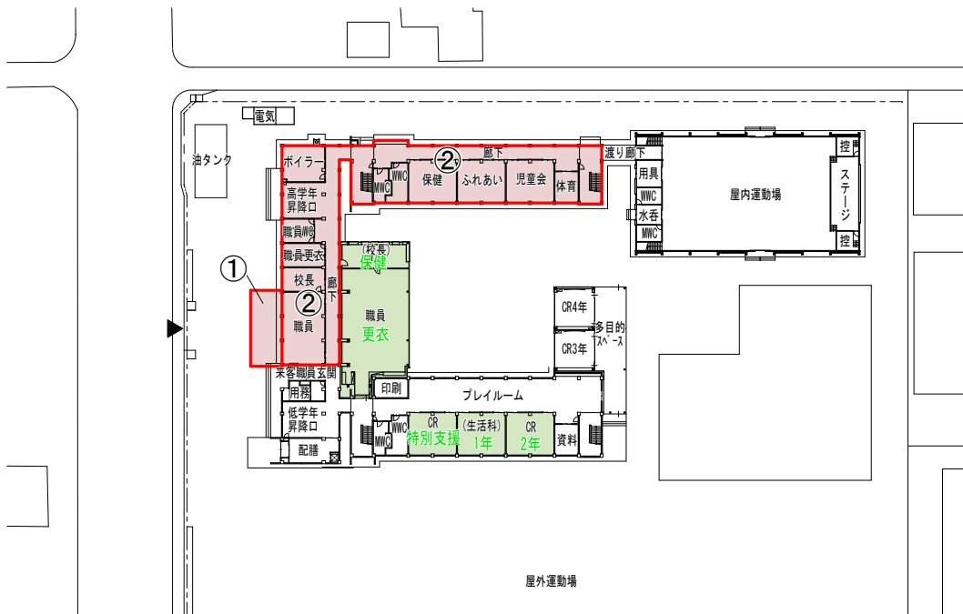
配置・1階計画図
