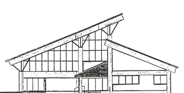
南側立面図
